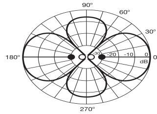
Figure 3.31 Doğrusal dört kutuplu
