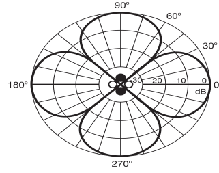
Figure 3.30 Yanal Dört kutuplu kaynak.
