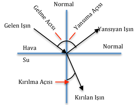
Figure 3.17 Yansıma ve kırılma dalga davranışı.
