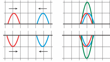
Figure 3.36 Örtüşünce artan (+), (-) Dalga pozisyonu.
