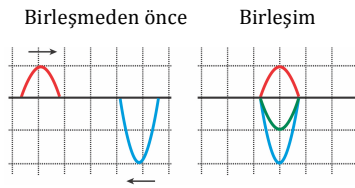
Figure 3. 27 Orantılı yıkıcı dalga birleşimi.
