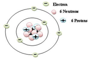
Figure 3.12 Artı ve eksi nötröl atomların davranışları.
