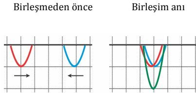
Figure 3.25 Negatif, yapıcı dalga birleşimi.
